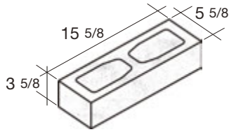
6x4x16 Quik-Brik®
