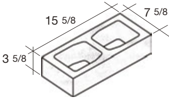
8x4x16 Quik-Brik®
