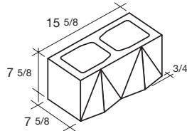
8x8x16 Hi-Lite Mark II
