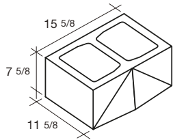
12x8x16 Hi-Lite Mark I
