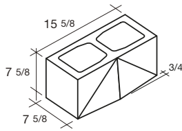
8x8x16 Hi-Lite Mark I
