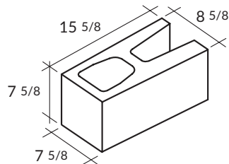
8x8x16 Facet Open End
